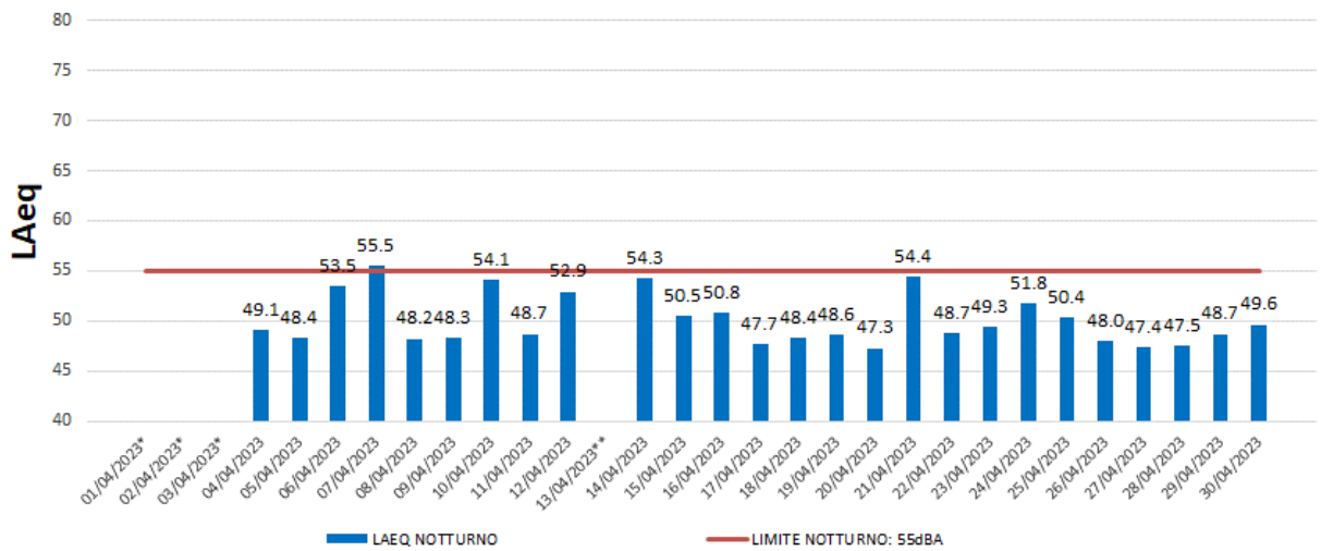
STAZIONE DI MISURA FCOPTO02: LAEQ GIORNALIERO NOTTURNO
