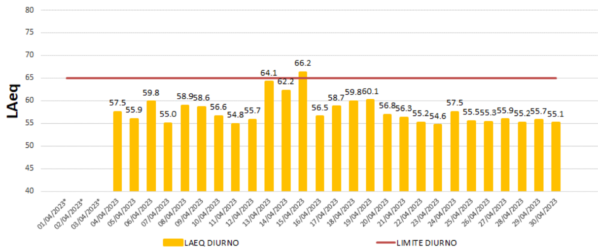
STAZIONE DI MISURA FCOPTO02: LAEQ GIORNALIERO DIURNO
