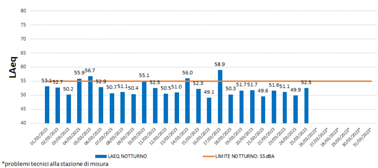
STAZIONE DI MISURA FCOPTO001: LAEQ GIORNALIERO NOTTURNO
