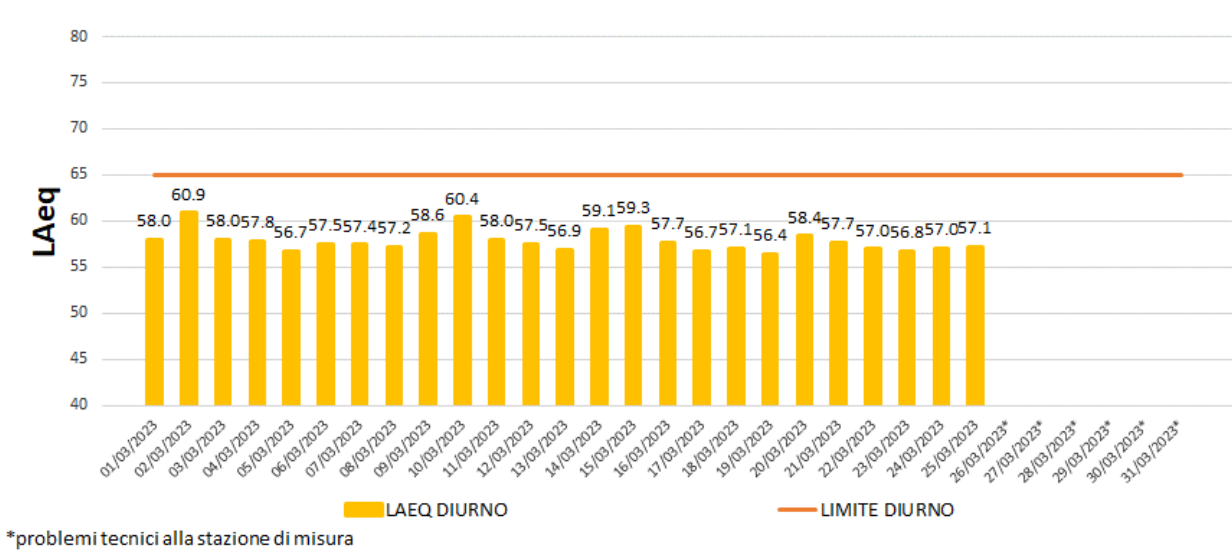
STAZIONE DI MISURA FCOPTO001: LAEQ GIORNALIERO DIURNO
